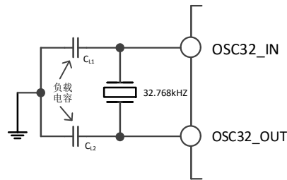
图 3-7 低速外部晶体电路
