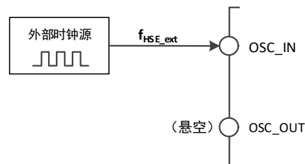
图 3-6 高速时钟源电路
