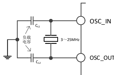
图 3-5 高速外部晶体电路
