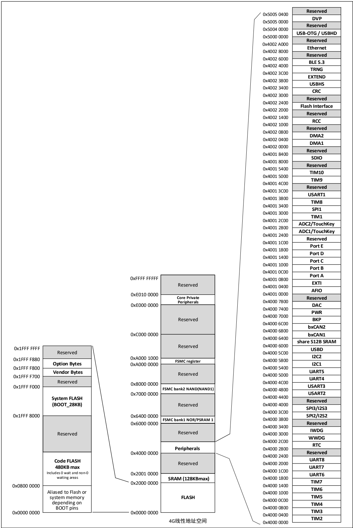
图 1-3 存储映像
