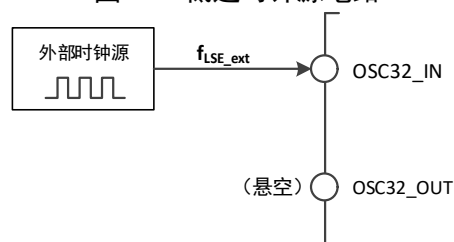
图 3-8 低速时钟源电路
