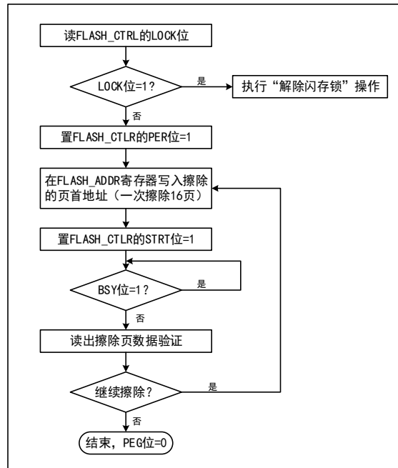
图 32-2 FLASH 页擦除
