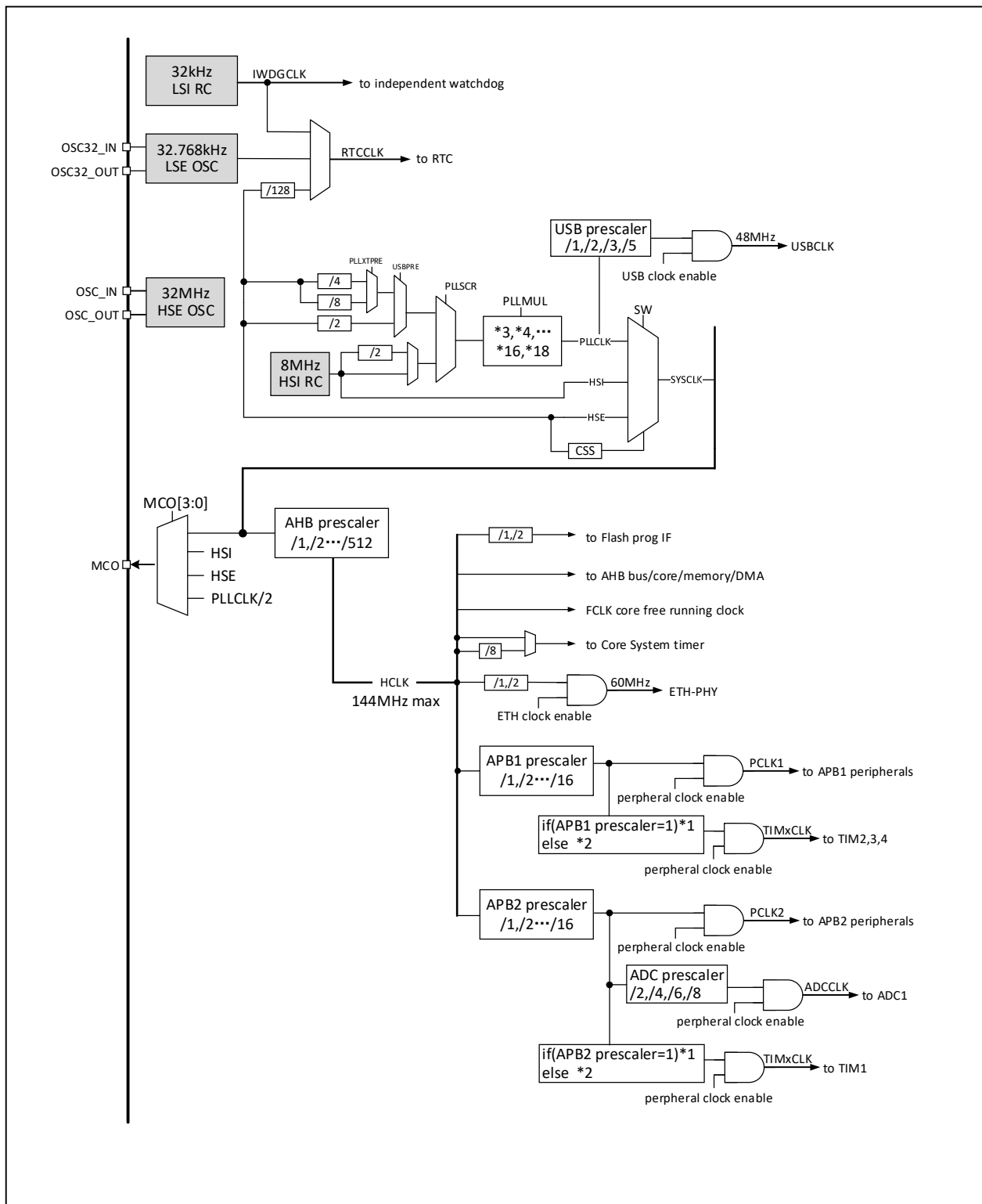
图 3-4 CH32FV208 时钟树结构
