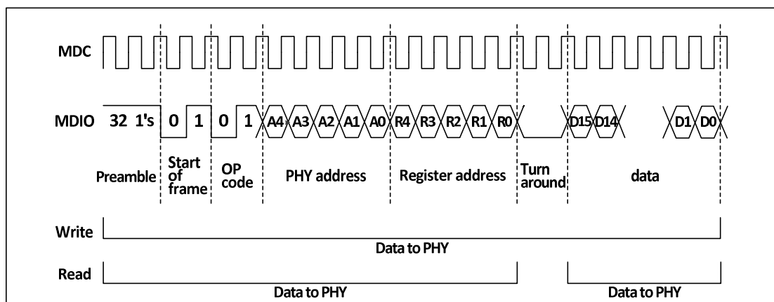
图 27-3 SMI 接口读写时序图
