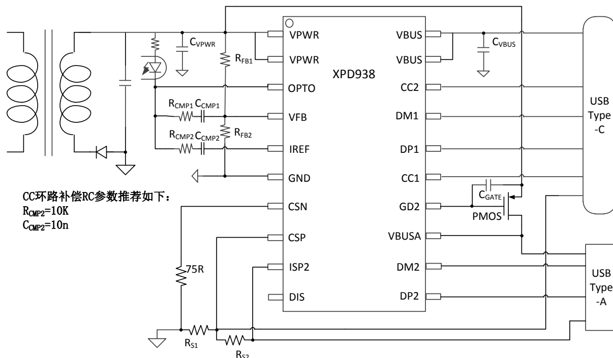
AC-DC应用图
