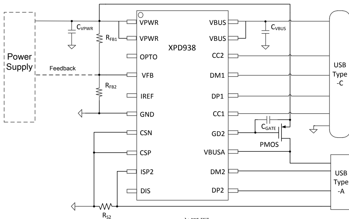
DC-DC应用图
