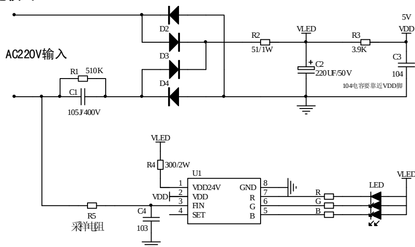
AC220V 阻容降压供电模式外围元件参数配置--参考:
