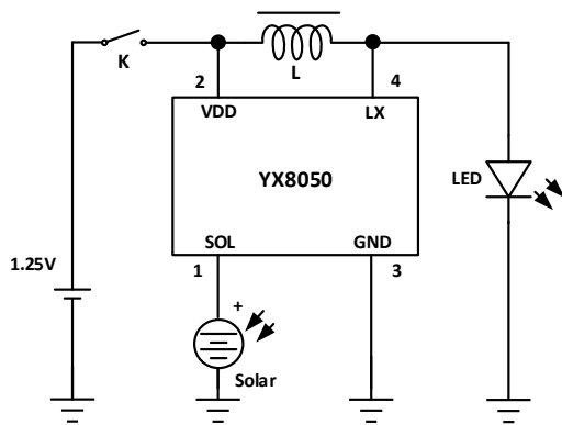
图 5. 推荐接法 1
