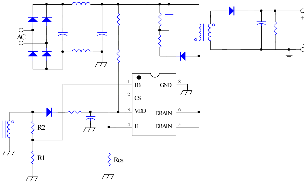
图 2.典型应用图
