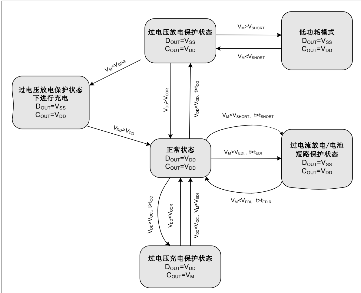
图-4 VA7071B 各状态之间的转换图
