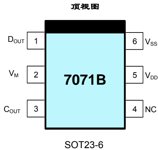
图-2 VA7071B 管脚排列 (不成比例)
