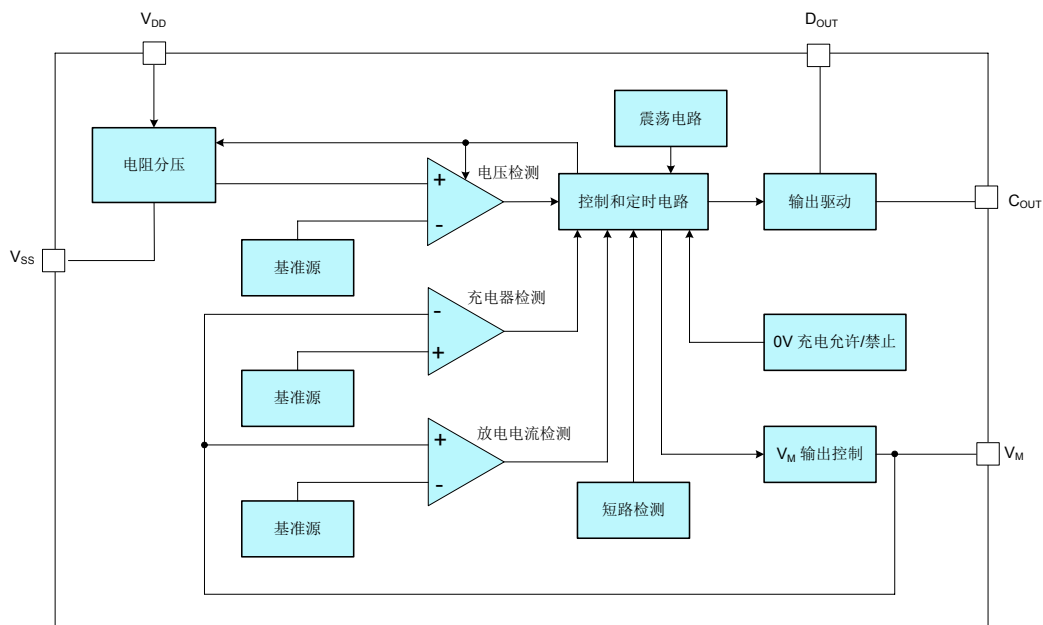
图-1 VA7071B 功能框图
