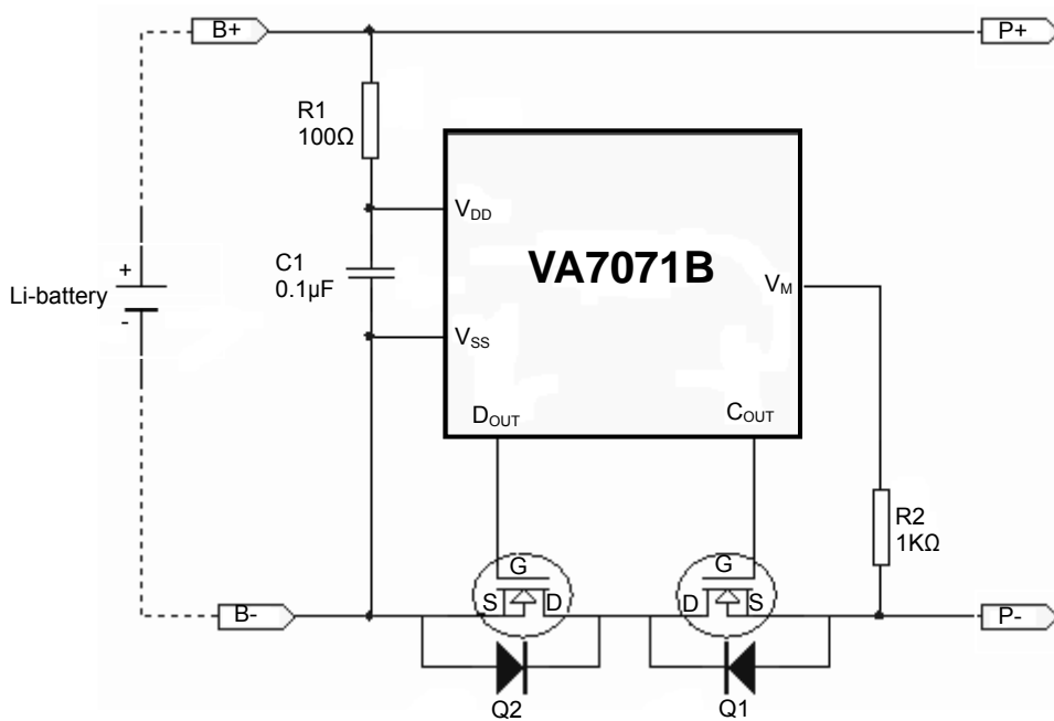
图-3 VA7071B 典型应用电路图
