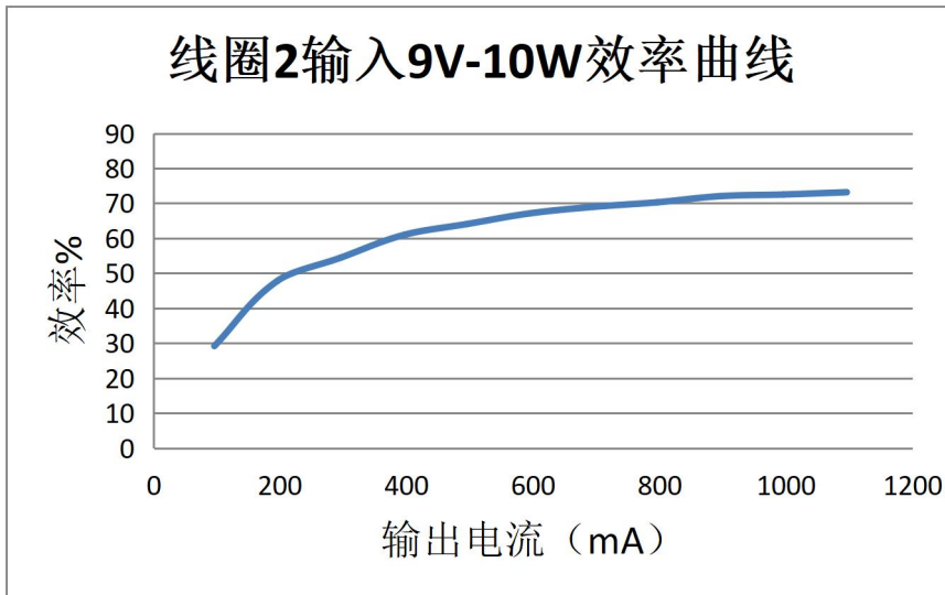
图 18 线圈 2 带载 10W 效率 (使用 IDT P9221_R RX)
