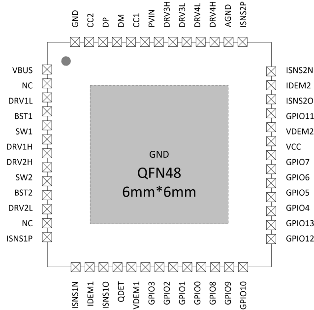
图 2 IP6862 引脚图
