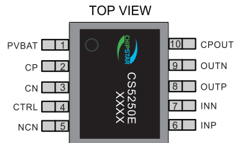
CS5250E(ESOP10 PACKAGE)
