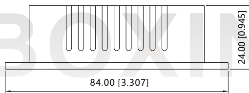
正视图
