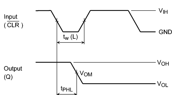
Fig. 12.8.2 t_{PHL} , t_w
