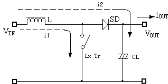
开关式 DC/DC 升压转换器工作原理图
