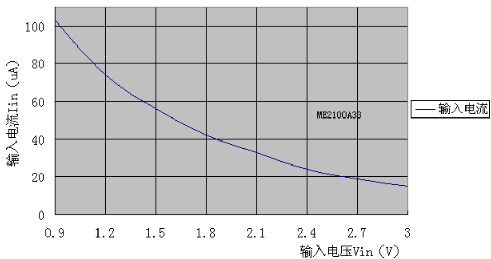
输入电压VS. 输入电流 Topr=25°C
