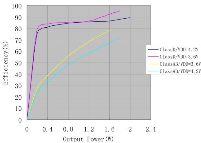
(3) 效率与输出功率曲线(R L =4Ω)
