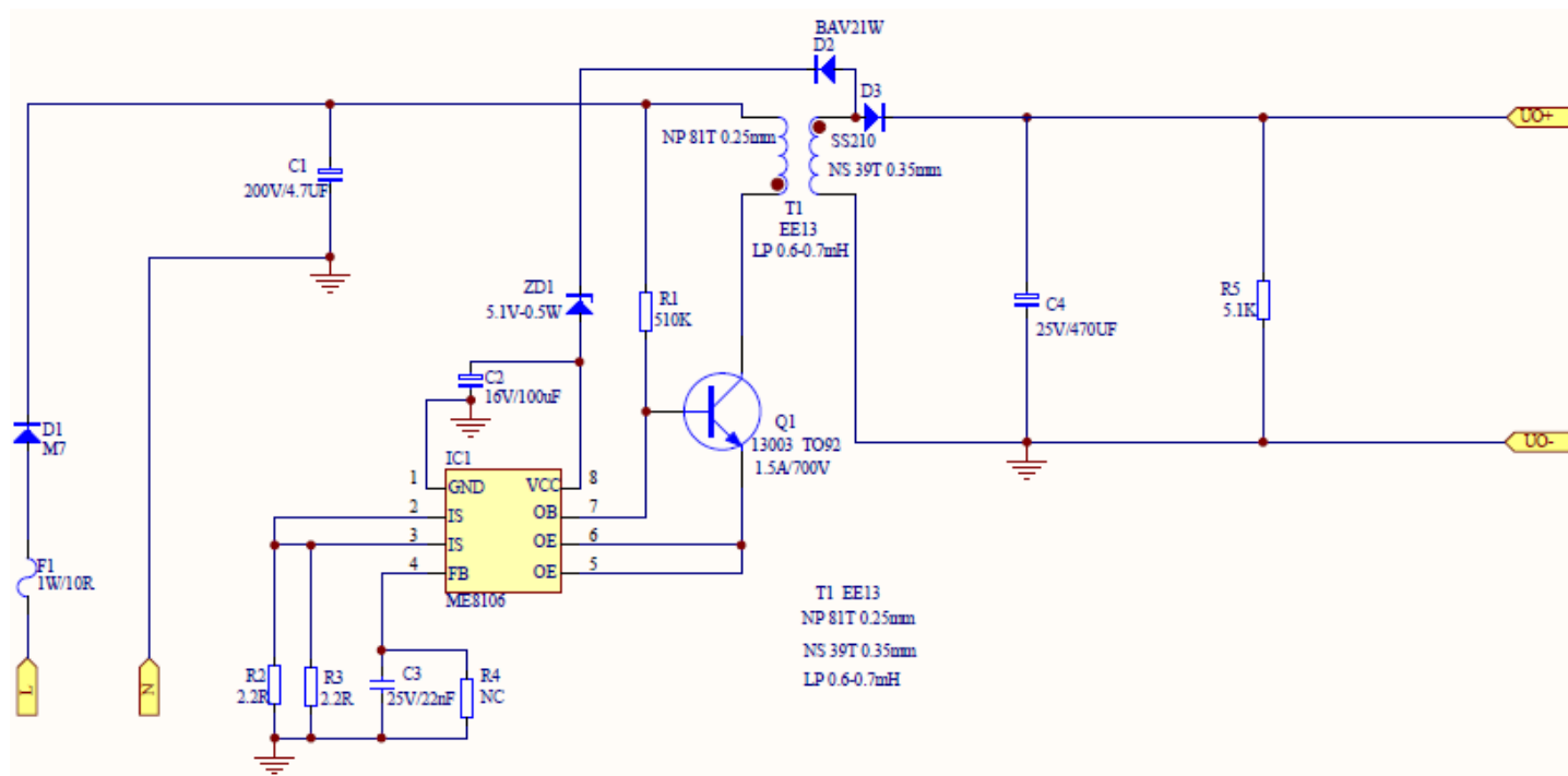
图.1 ME8106 典型应用电路
