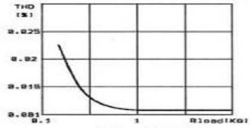
失真 vs 负载电阻
