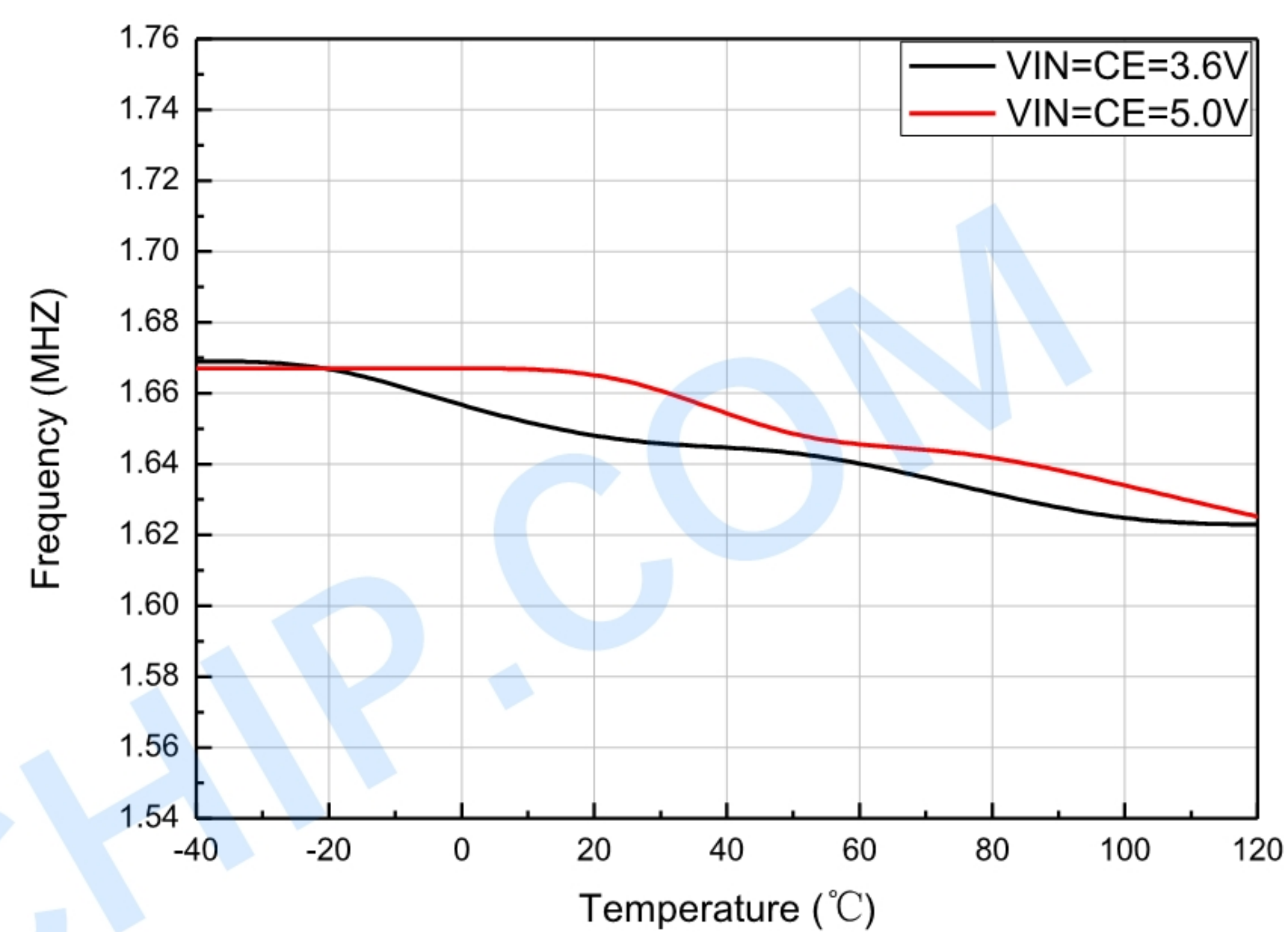
频率温度曲线
