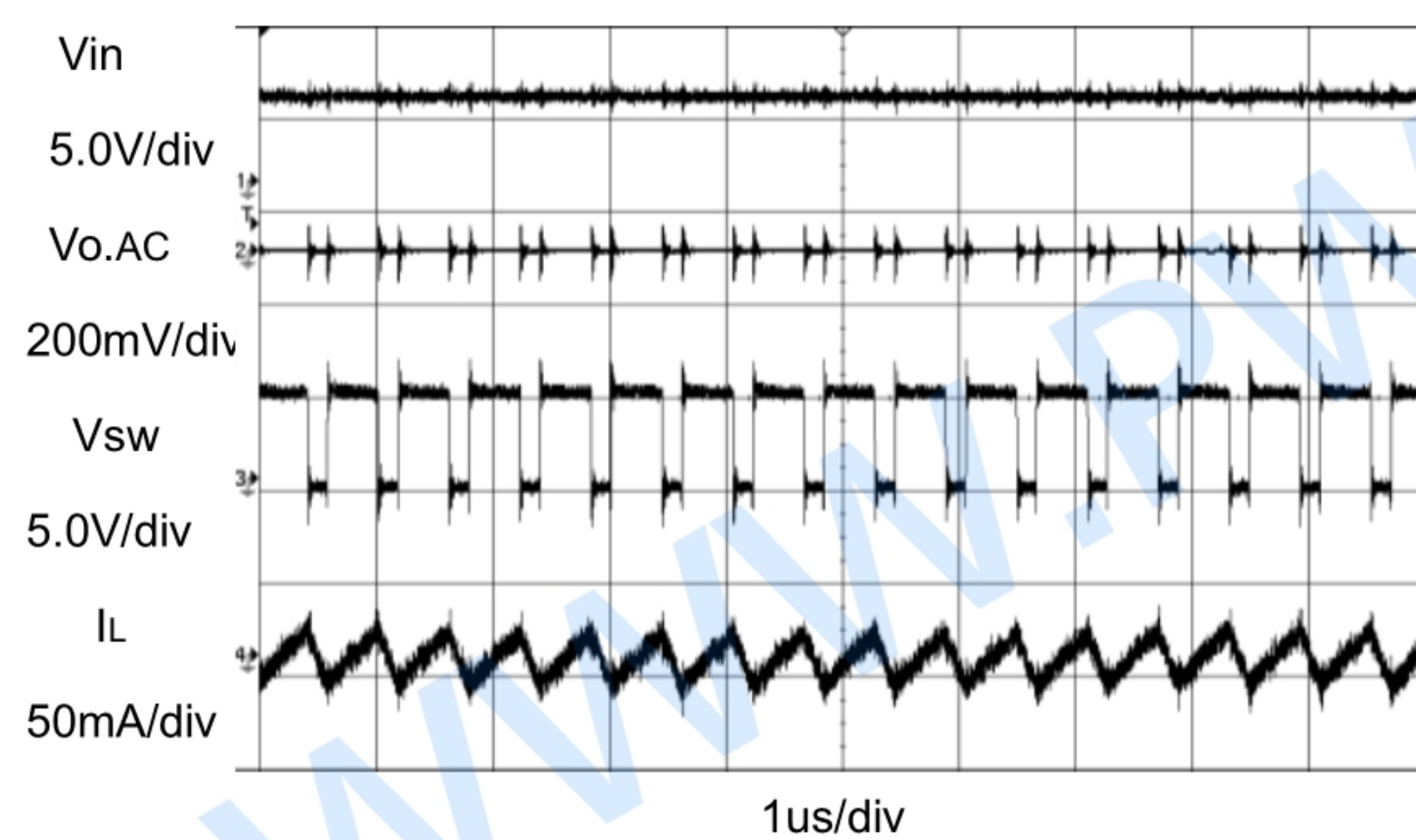
中等负载波形
