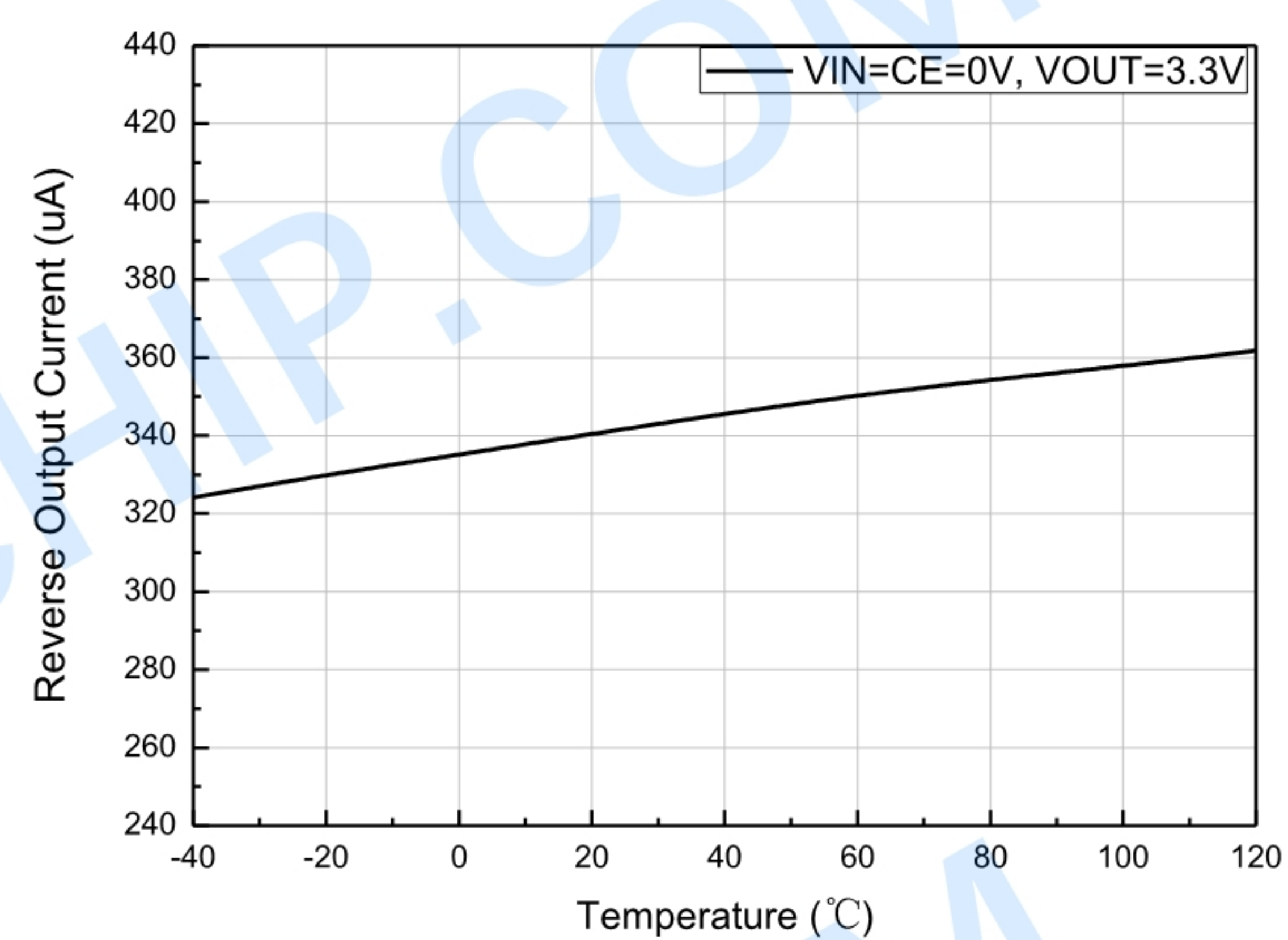
反向输出电流温度曲线
