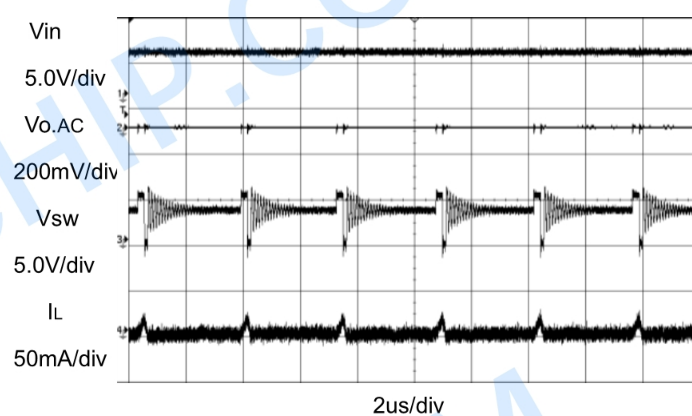
轻载波形
