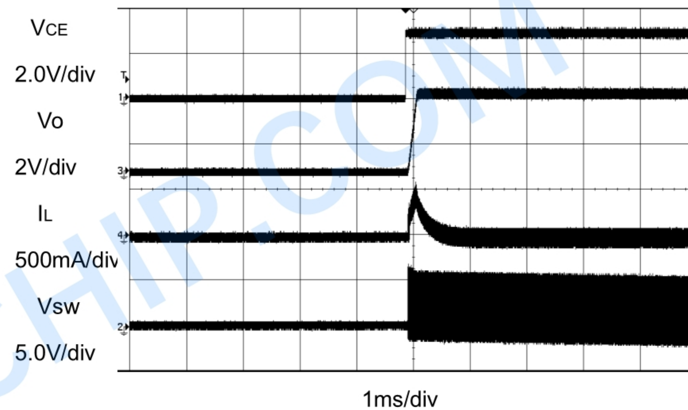
CE 开启
