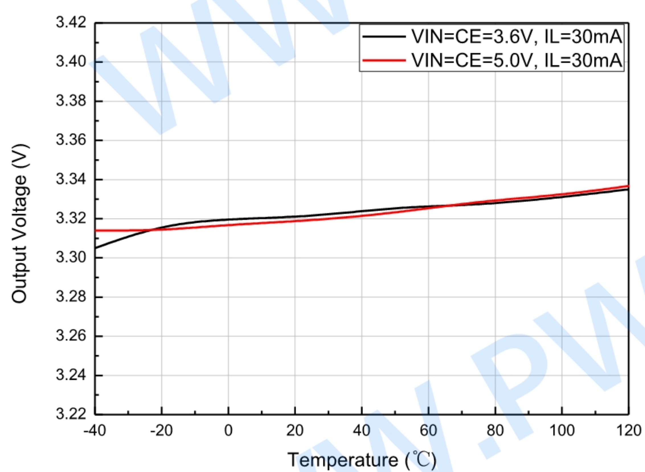
输出电压温度曲线
