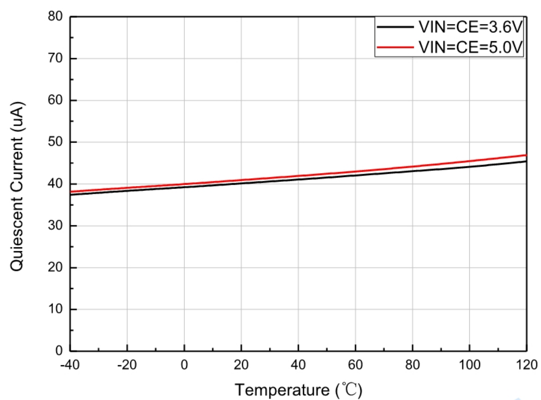
静态电流温度曲线
