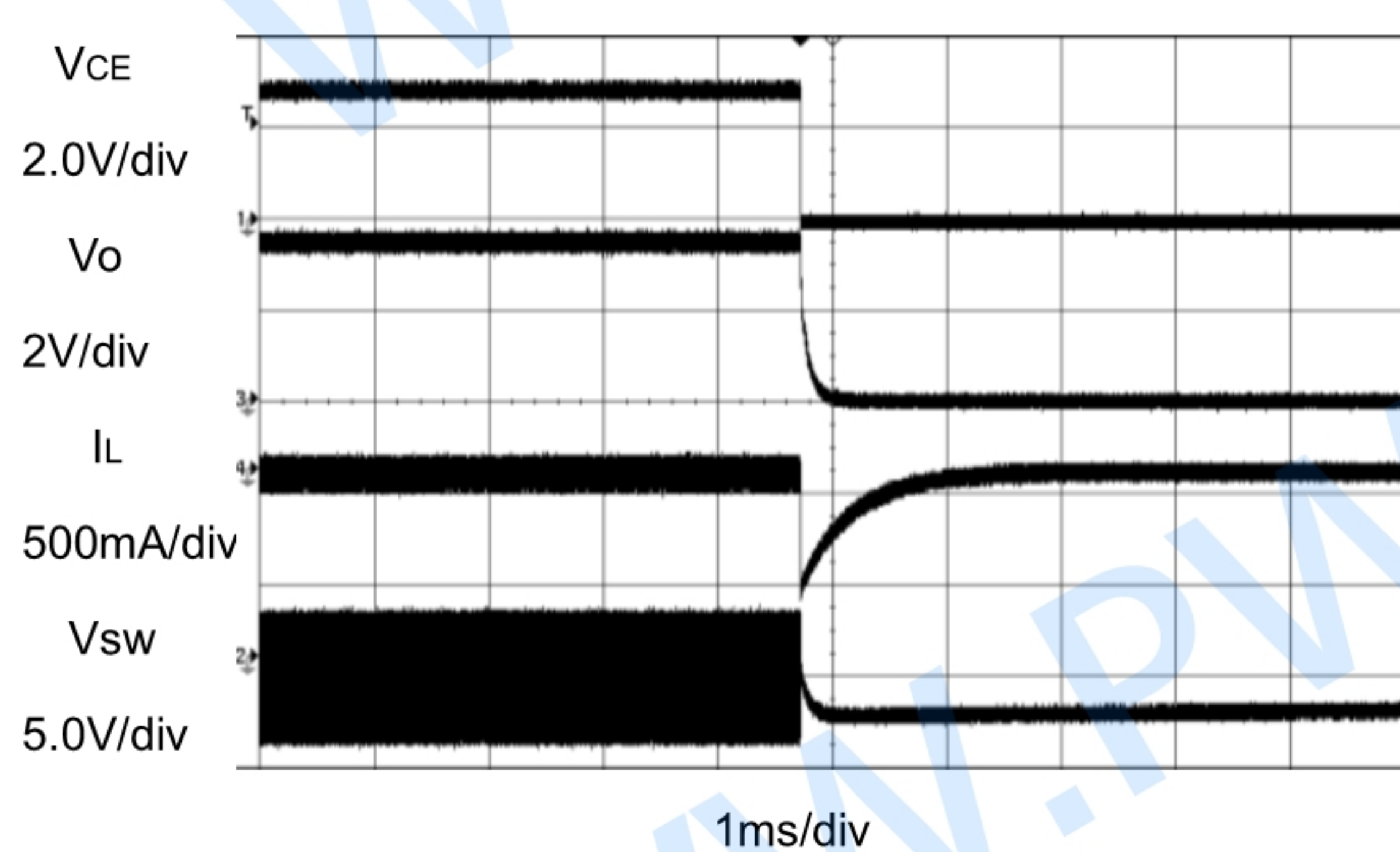
CE 关断
