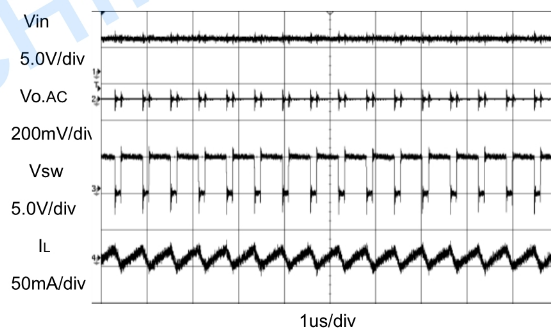
重载波形
