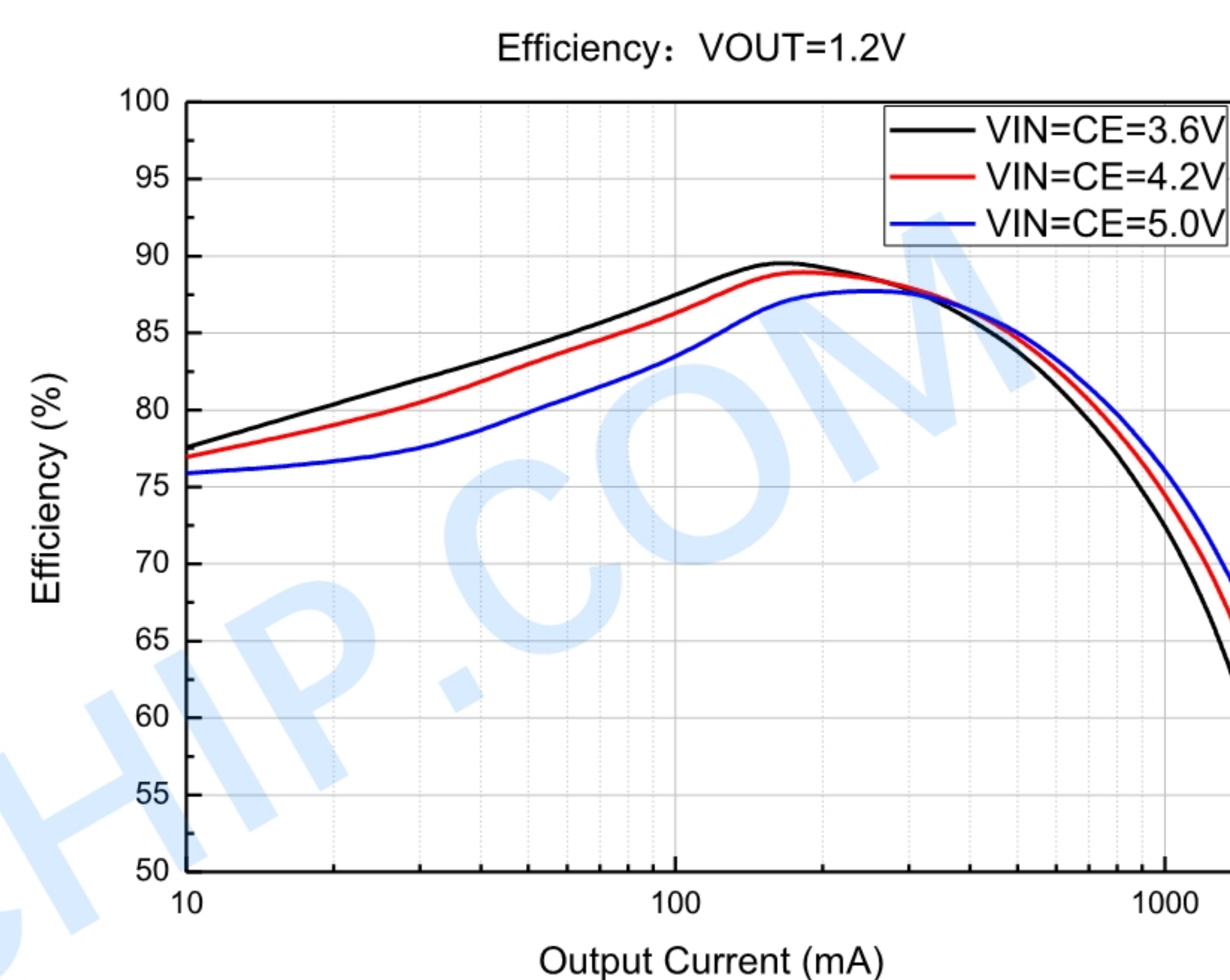
效率 @ VOUT=1.2V
