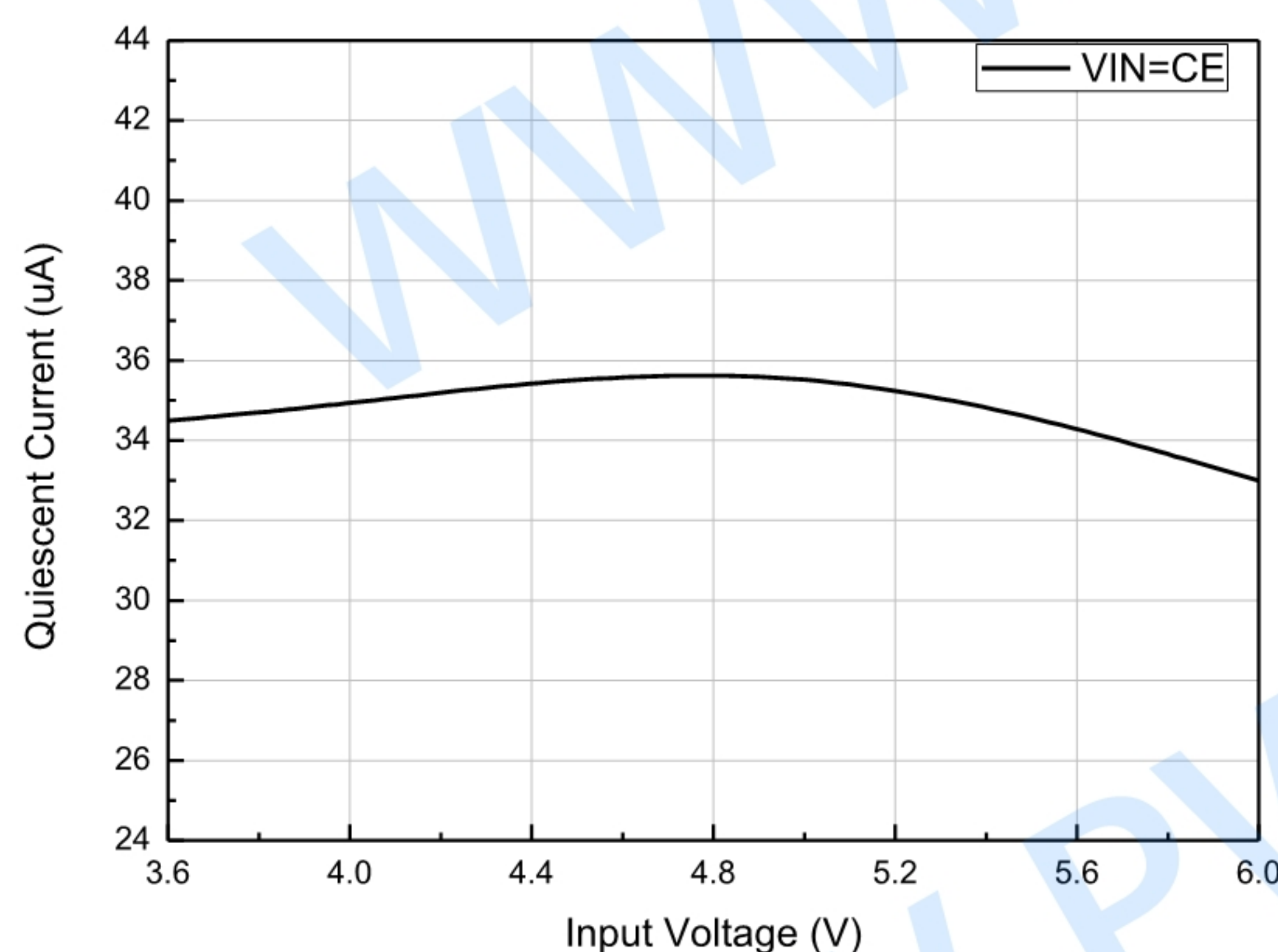
静态电流 Vs. 输入电压
