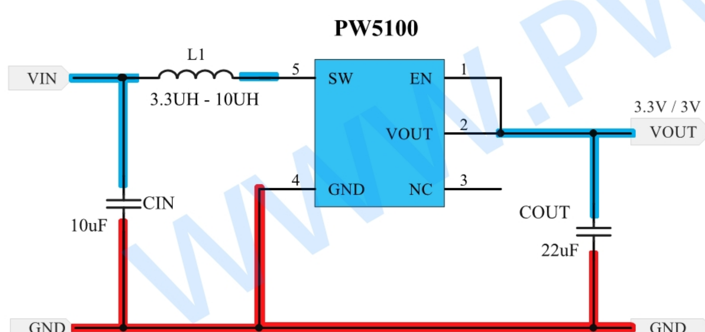
图 1：典型应用电路图 3.3V 和 3V
