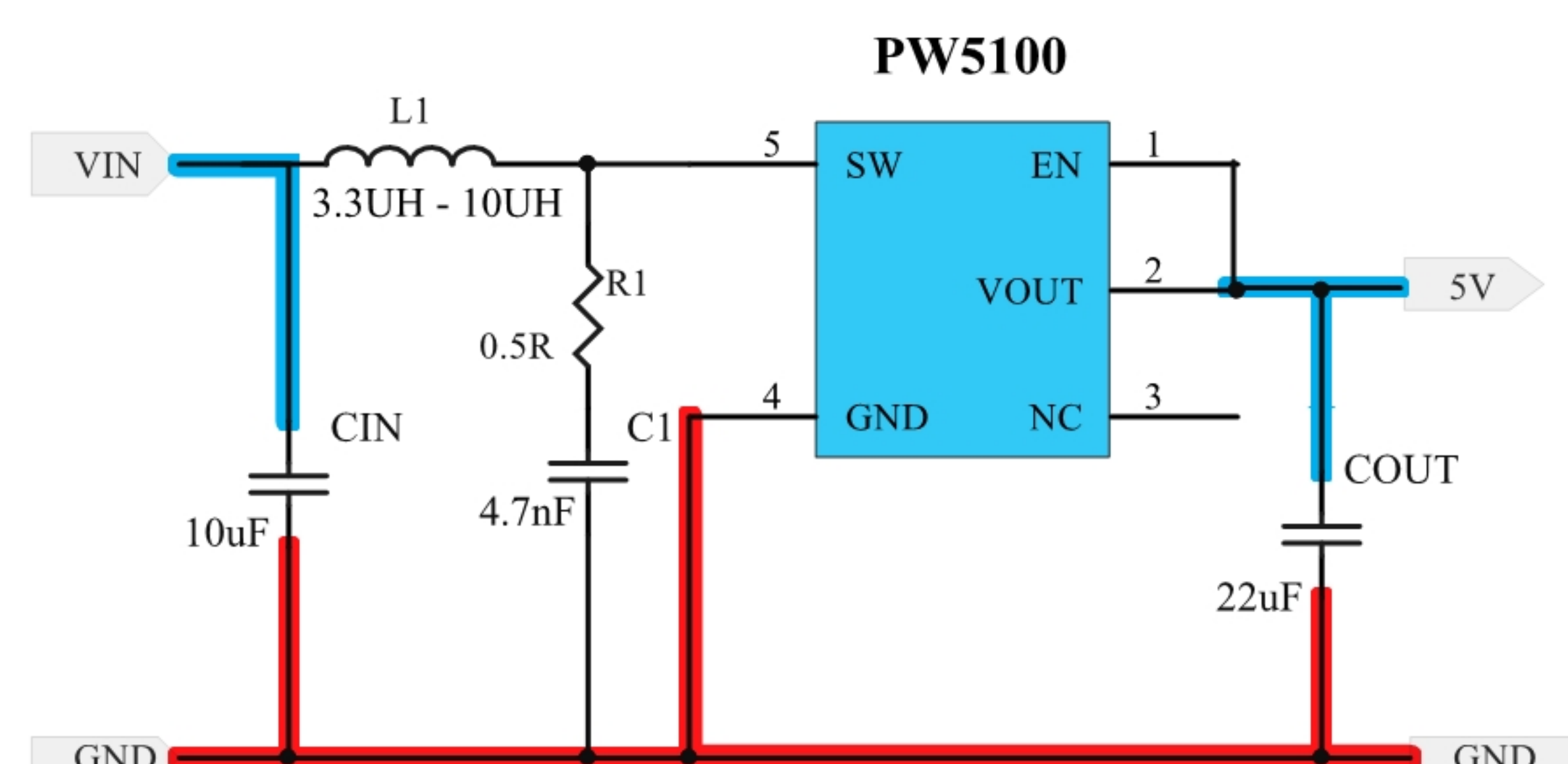
图 2：典型应用电路图：5V（增加R1和C1，吸收尖峰，容易过EMI） R1,C1可以用0603封装。
