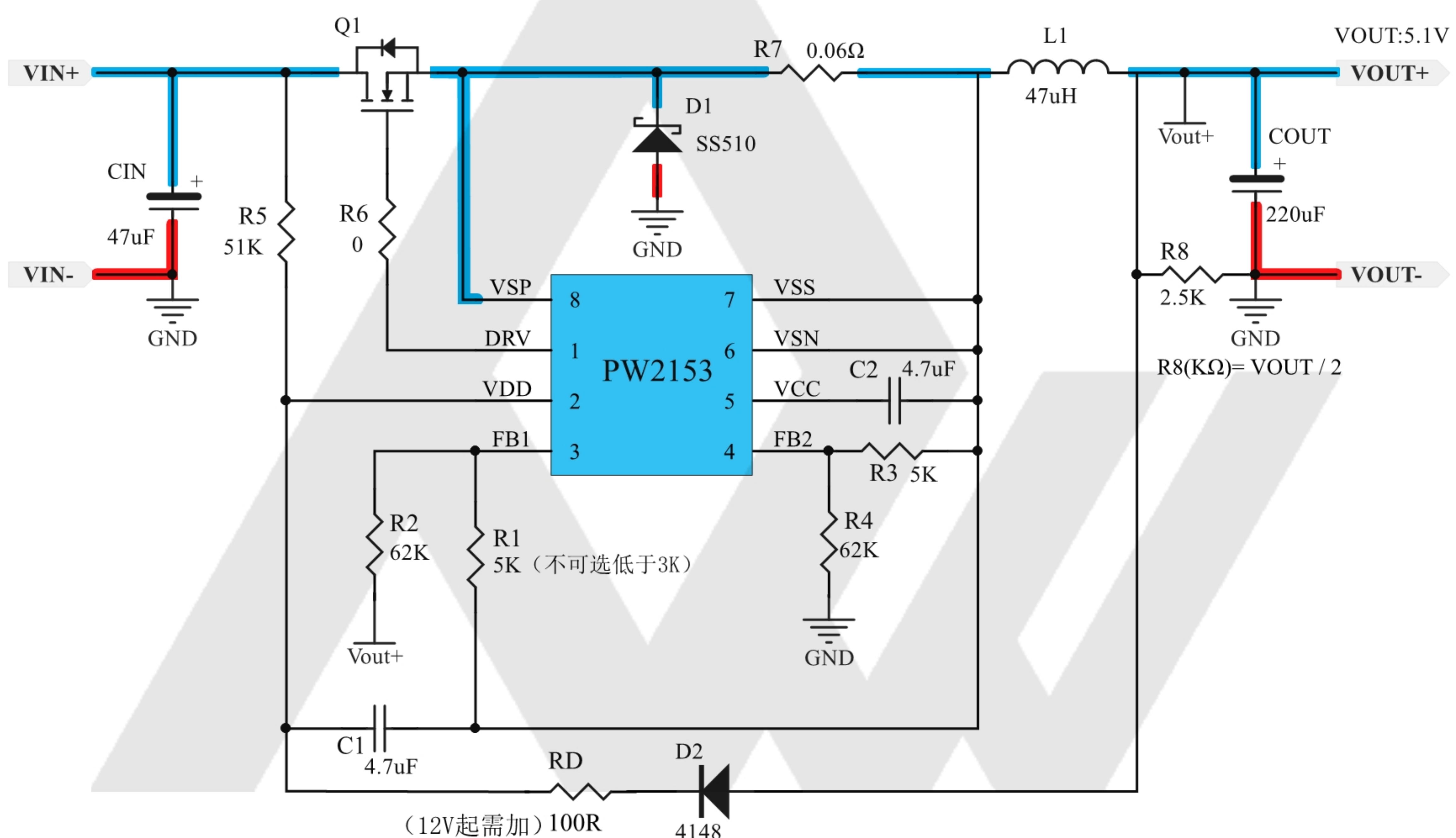
典型应用电路图：Vout: 5.1V
