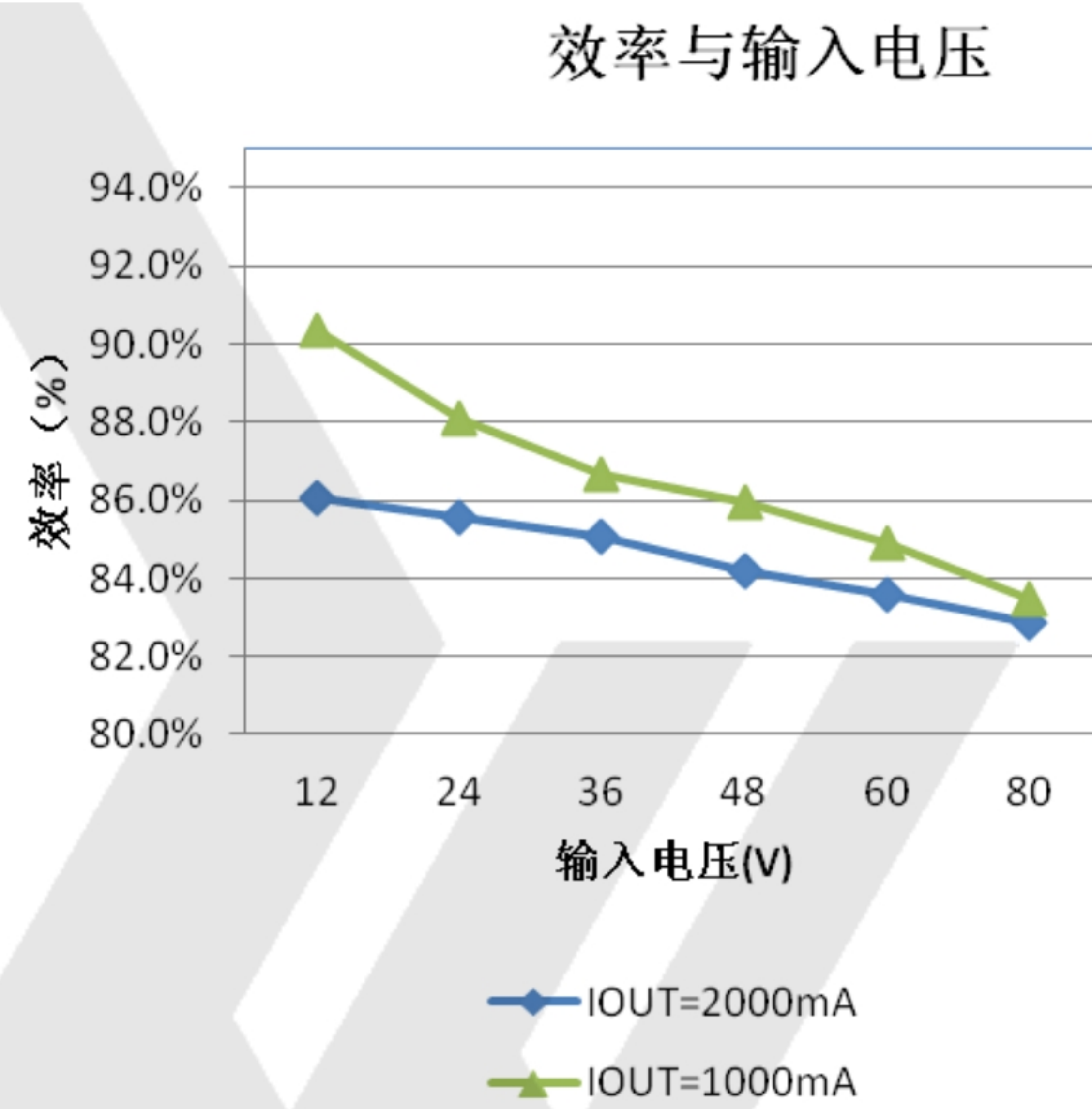
效率与输入电压及输出电流特性曲线(Vout=5V)
