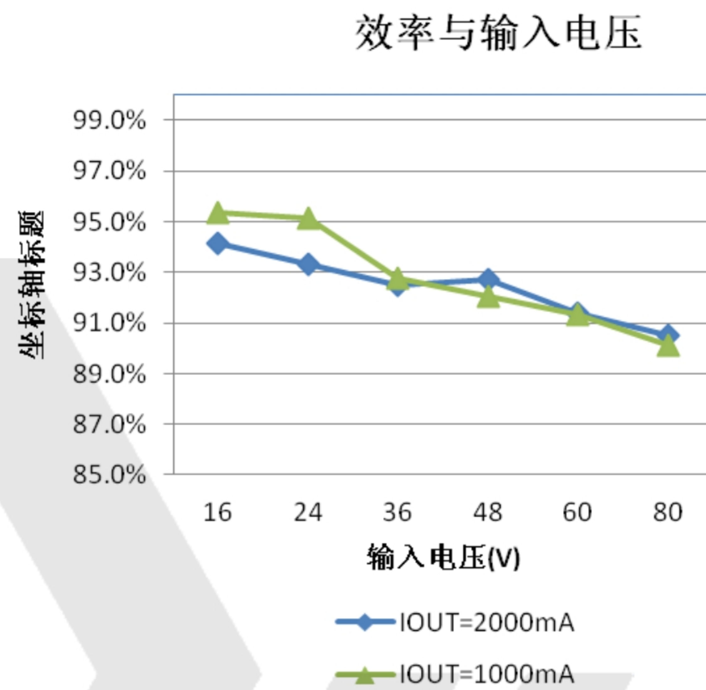
效率与输入电压及输出电流特性曲线(Vout=12V)
