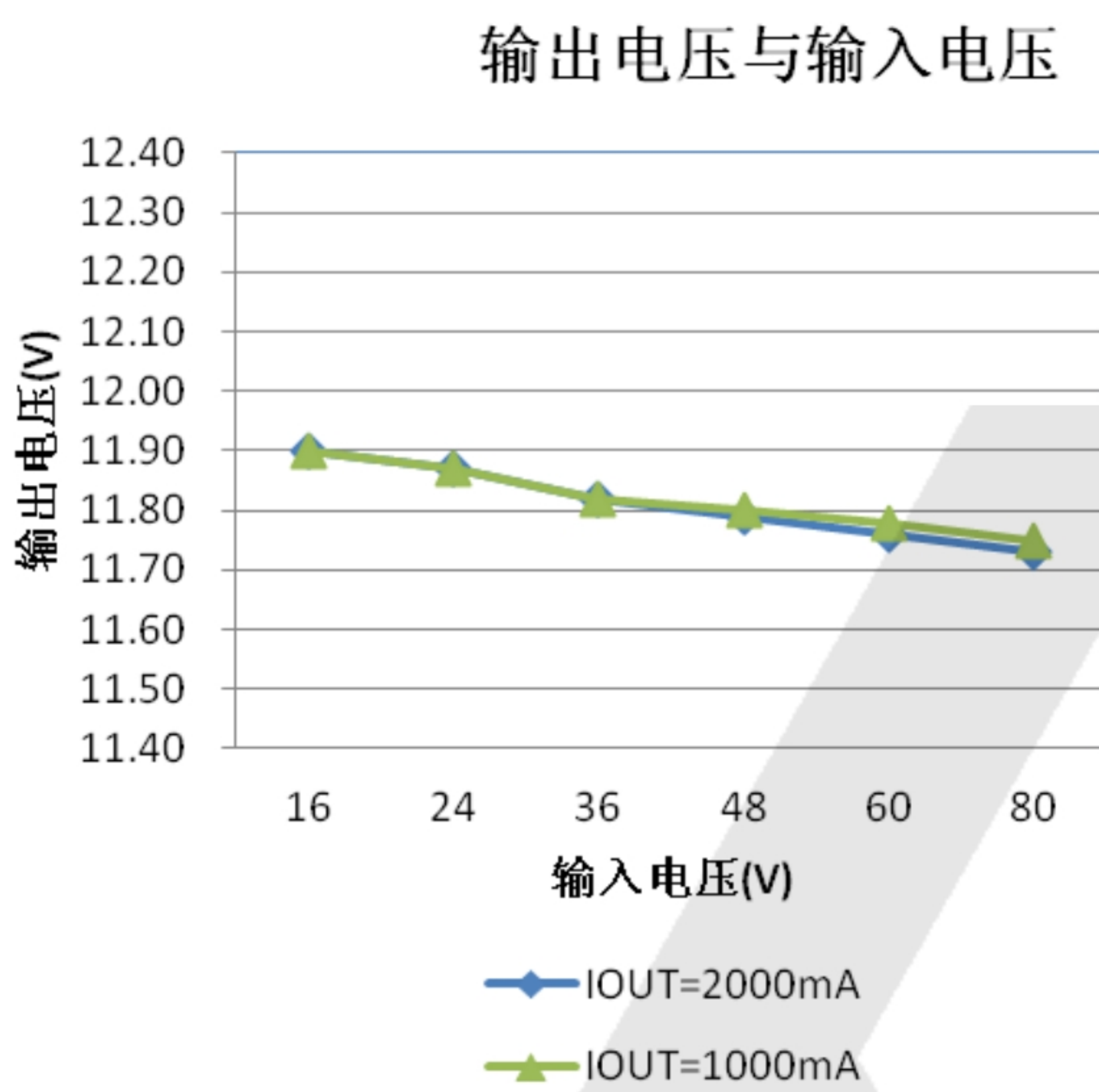
12V 输出电压与输入电压及输出电流特性曲线
