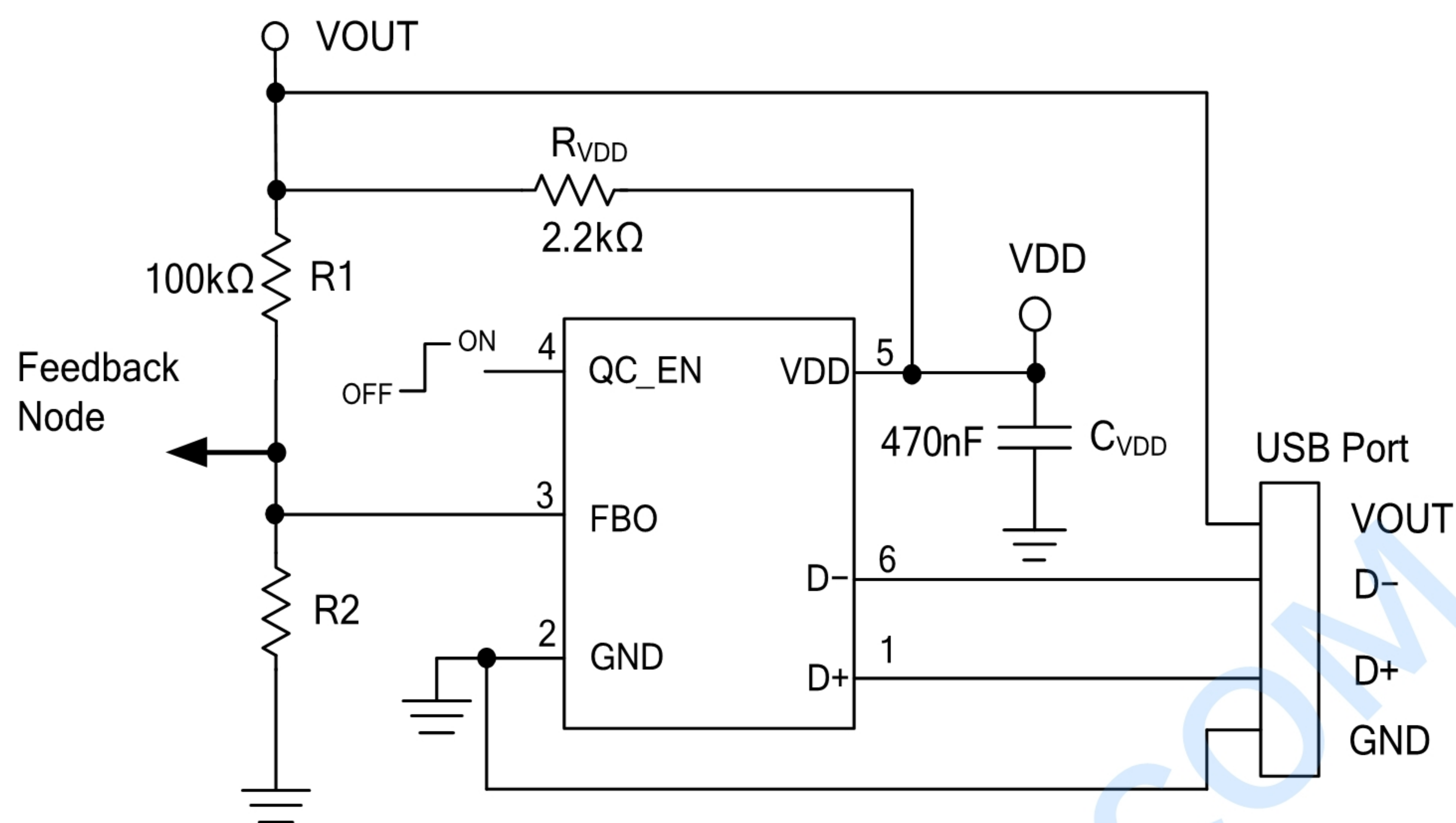
典型的应用原理图 1
