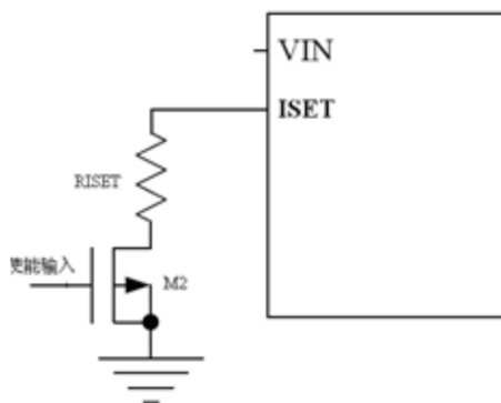
图 5. PL4056 的使能设计
