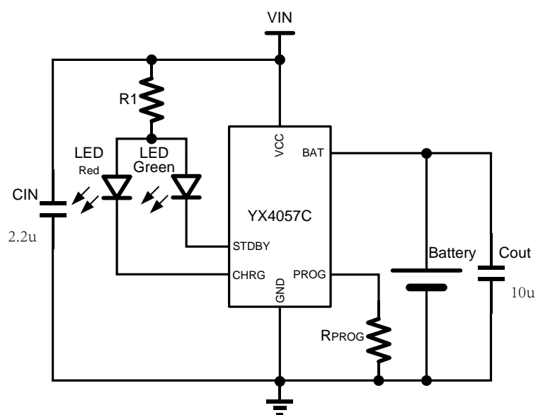
图 4. 典型应用电路
