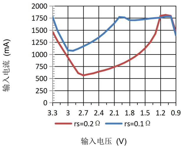
输入电压 (V) 输入电流 vs. 输入电压
