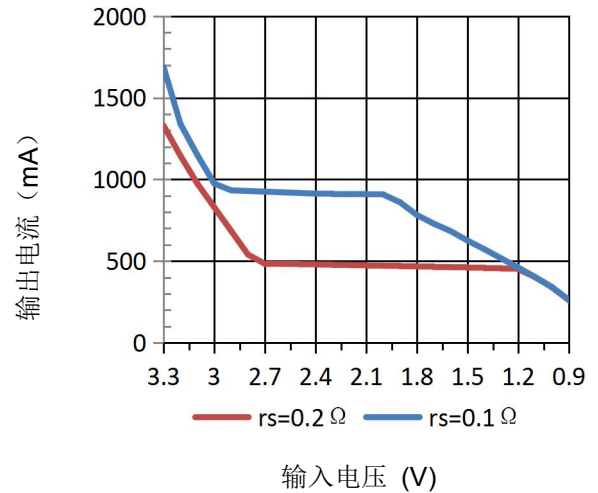
输入电压 (V) 输出电流 vs. 输入电压
